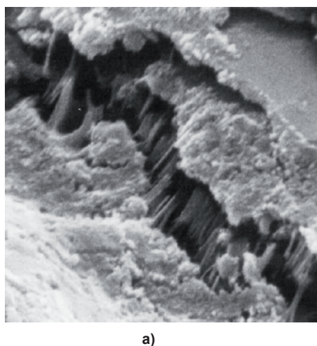
Rys. 8. Propagacja rys: a) PCC; b) beton cementowy (17)
