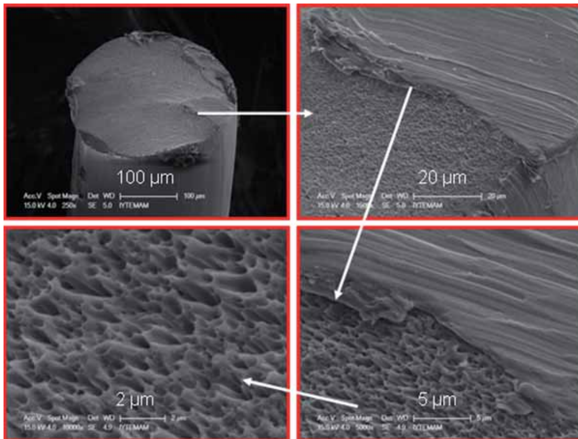
Rys. 1. Przekrój poręczny włókien stalowych pod elektronowym mikroskopem skaningowym
