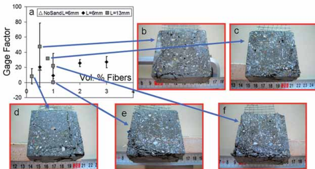
Rys. 17. a) Stała sensora w zależności od udziału objętościowego włókien. Przekroje poprzeczne próbek: b) mieszanka 5, c) mieszanka 10, d) mieszanka 9, e) mieszanka 7, f) mieszanka 6
