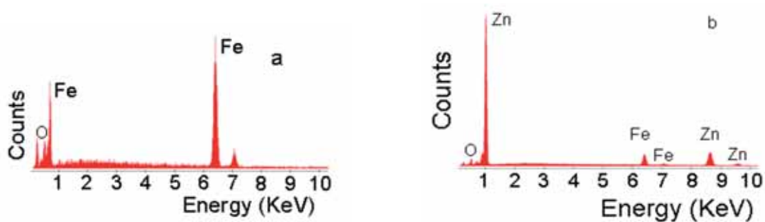
Rys. 4. Mikroanalizy rentgenowskie drutu siatki metalowej a) jądro, b) powierzchnia
