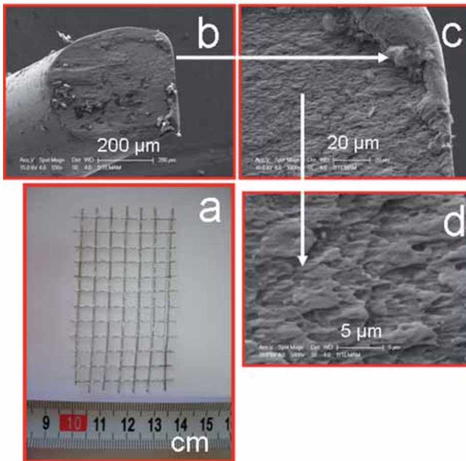
Rys. 3. Siatka metalowa a), przekrój drutu pod mikroskopem elektronowym b), warstwa powierzchniowa i jądro c), jądro drutu siatki d)
